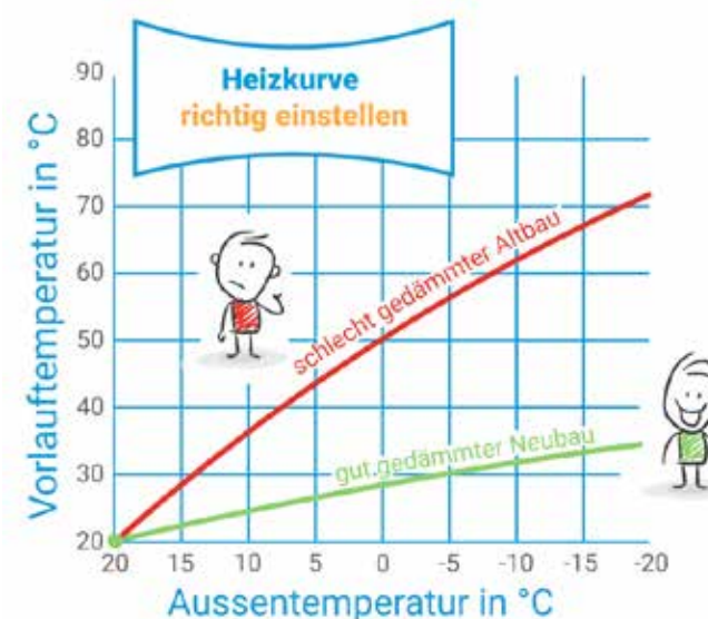
Abbildung 1: Heizkurve (Bildquelle: heizungsmacher.ch)
